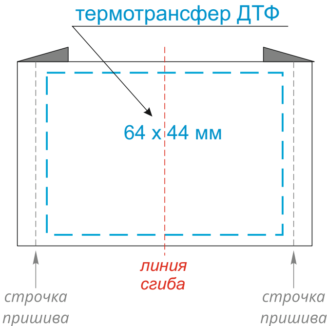
Лейбл пришивной тканевый 80 x 50 мм
